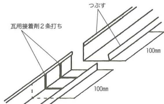
【 ジョイント部 】
