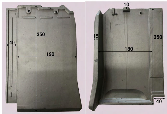
フラット調整瓦
