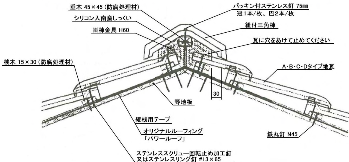
【 瓦が半端瓦で納まる場合 】
