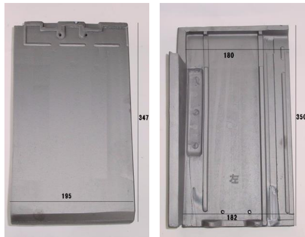
フラット半瓦
